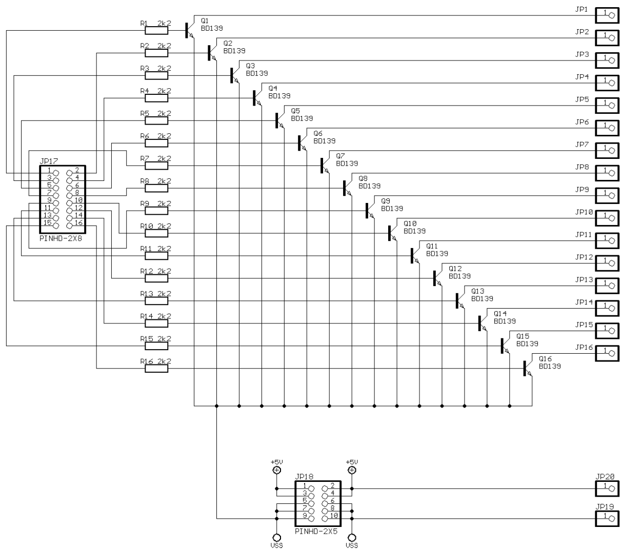
Schaltbild MTC64 Treiberplatine © 2002 by Doepfer Musikelektronik
